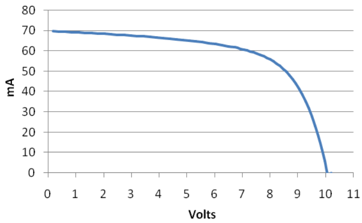
MP7.2-150 25% Sun
