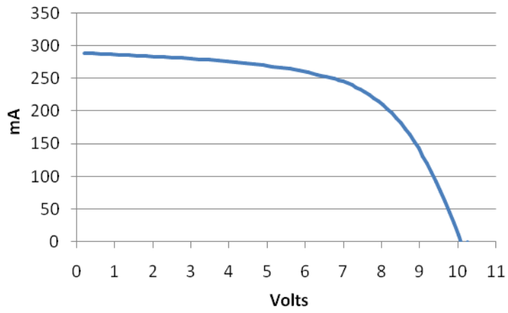
MP7.2-150 100% Sun
